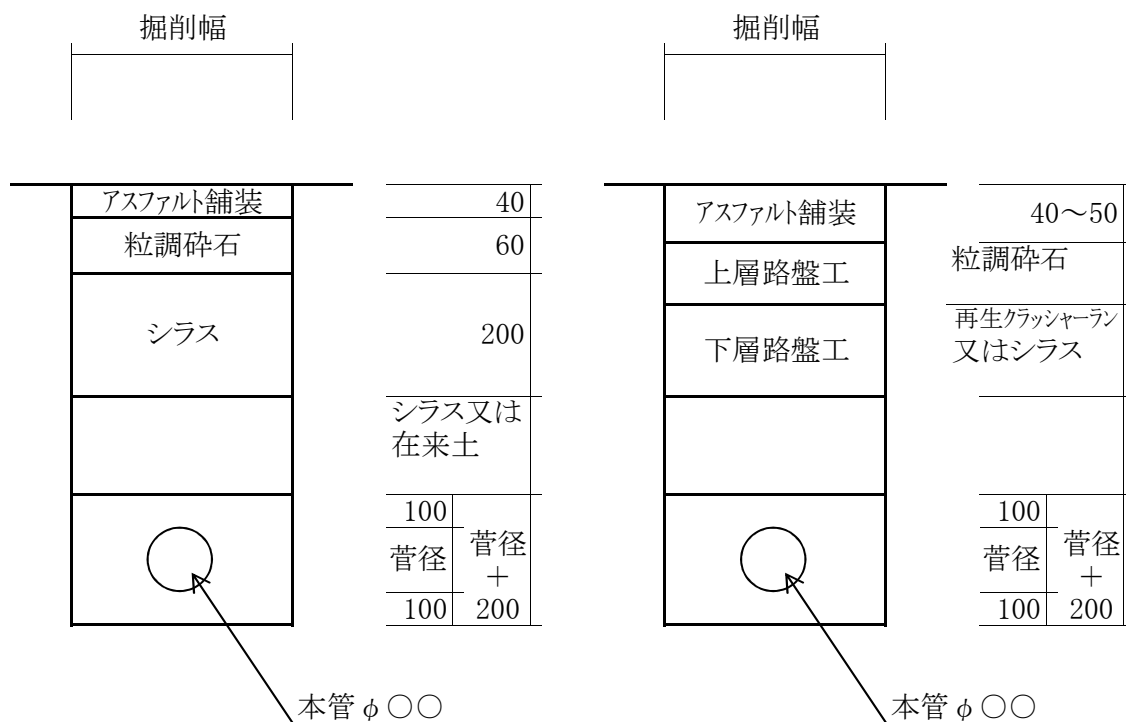
1) 標準舗装構成(一般道路) (単位:mm)
