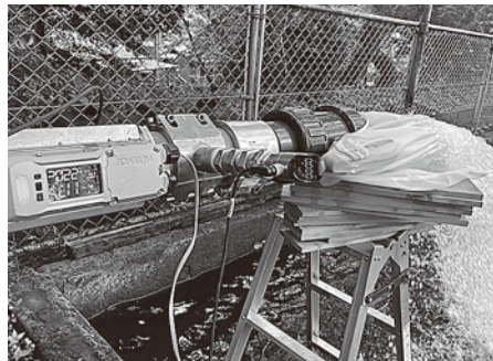
▲皇子原公園ポテンシャル測定
