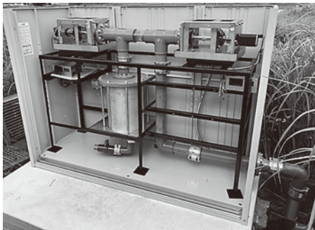
▲(参考) 狭野地区実証実験装置
