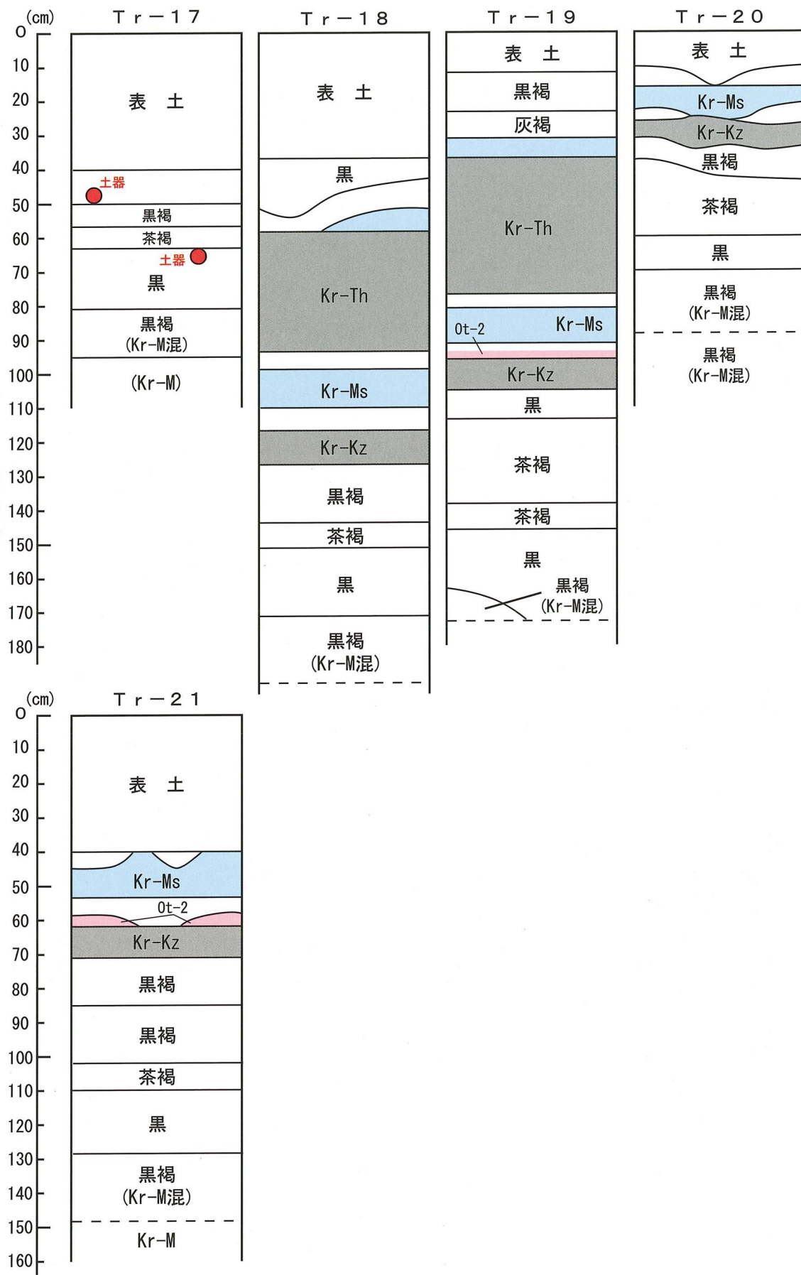
第8図 宇都地区試掘坑層序 (3)
