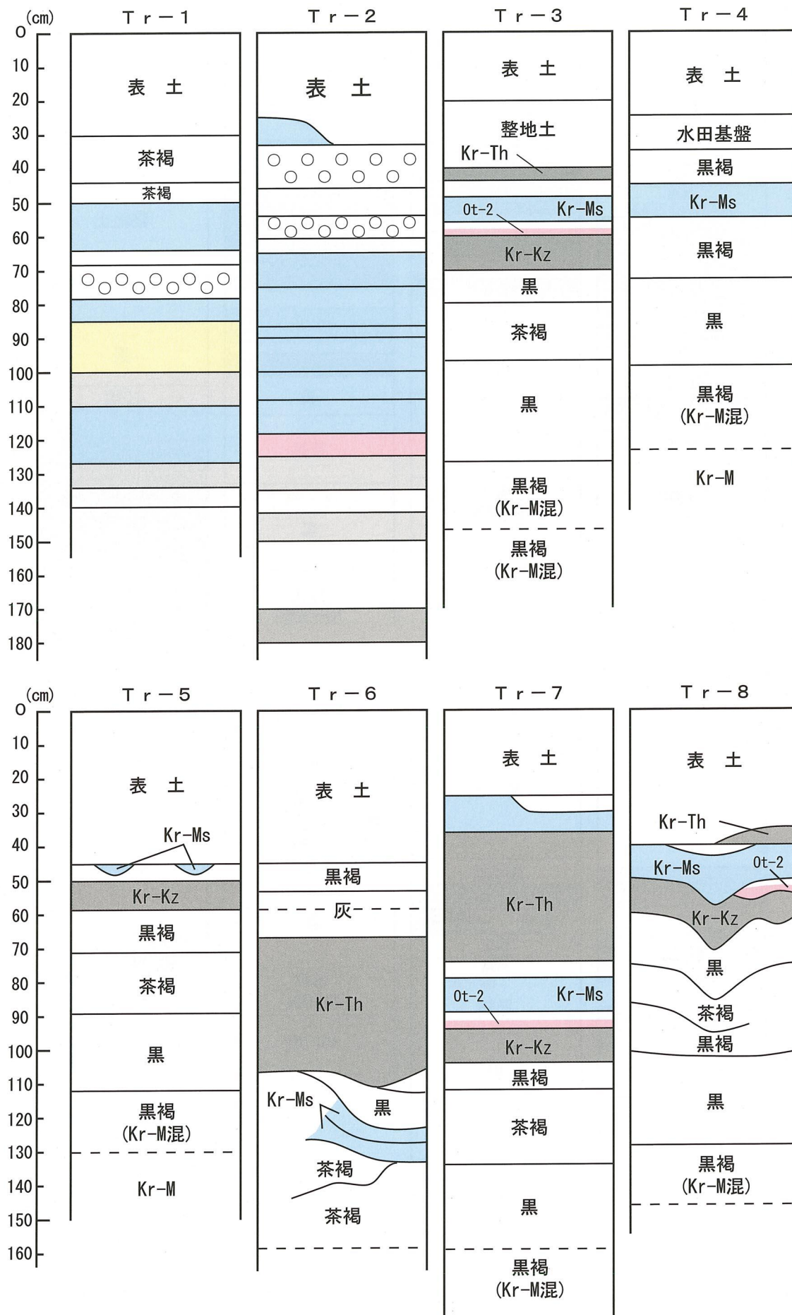
第6図 宇都地区試掘坑層序 (1)
