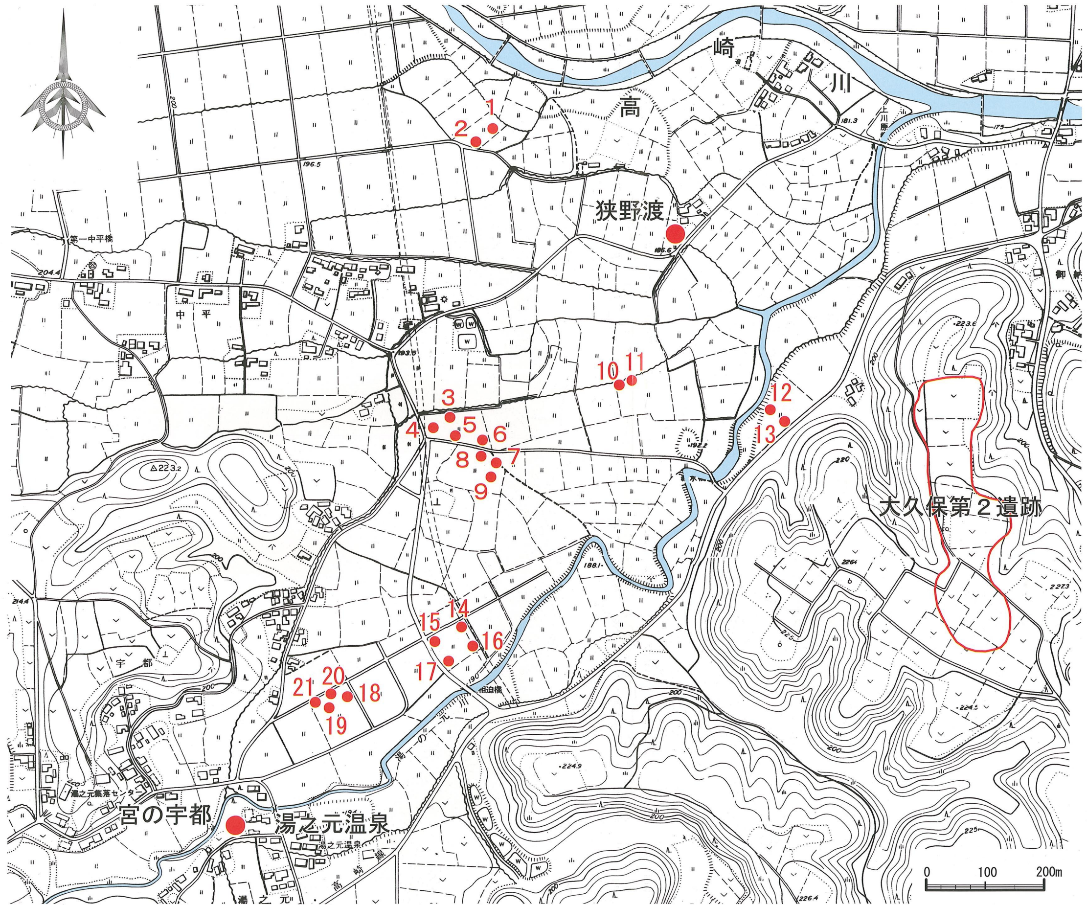
第5図 宇都地区試掘坑位置図
