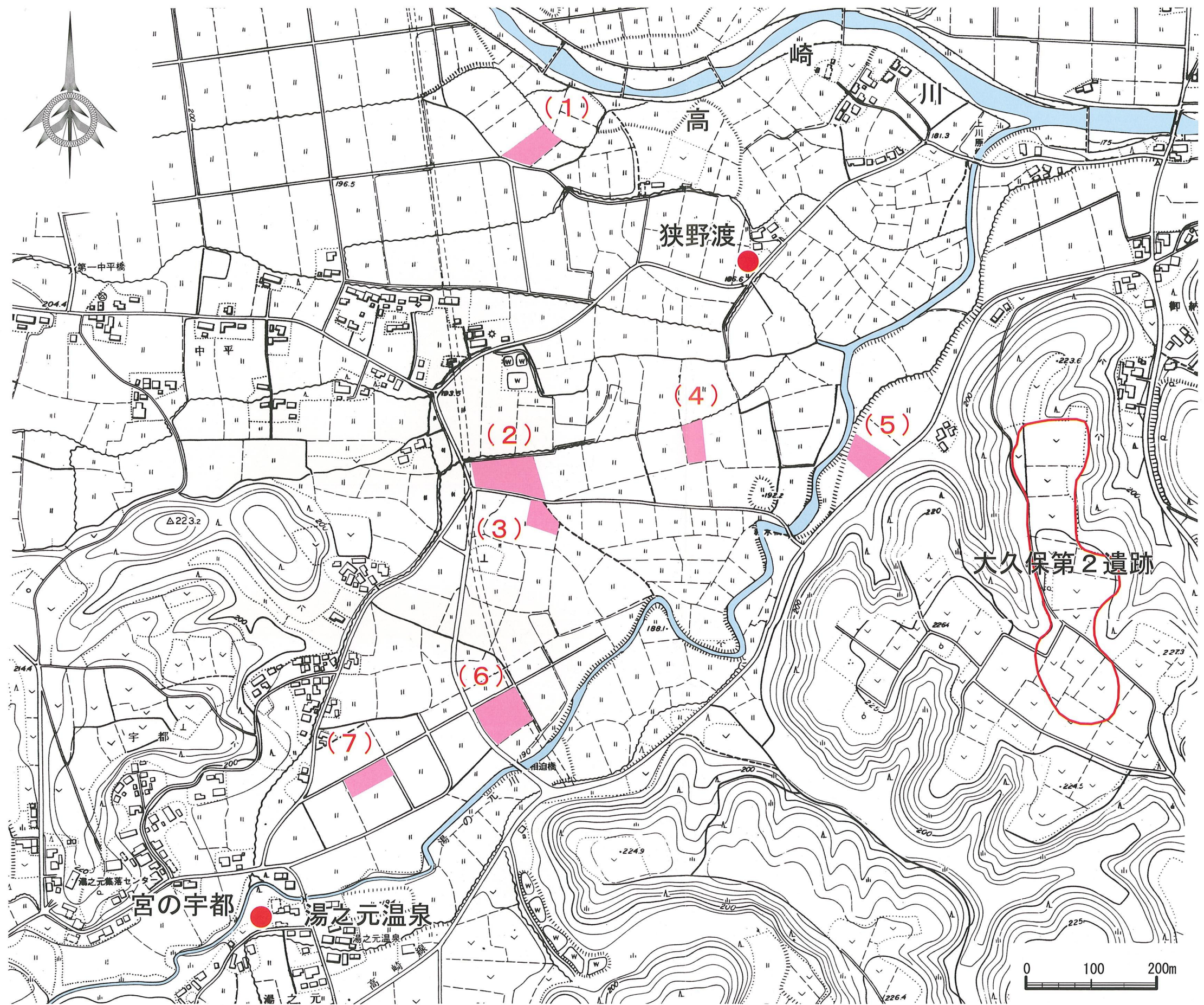
第4図 宇都地区試掘調査における地区位置図
