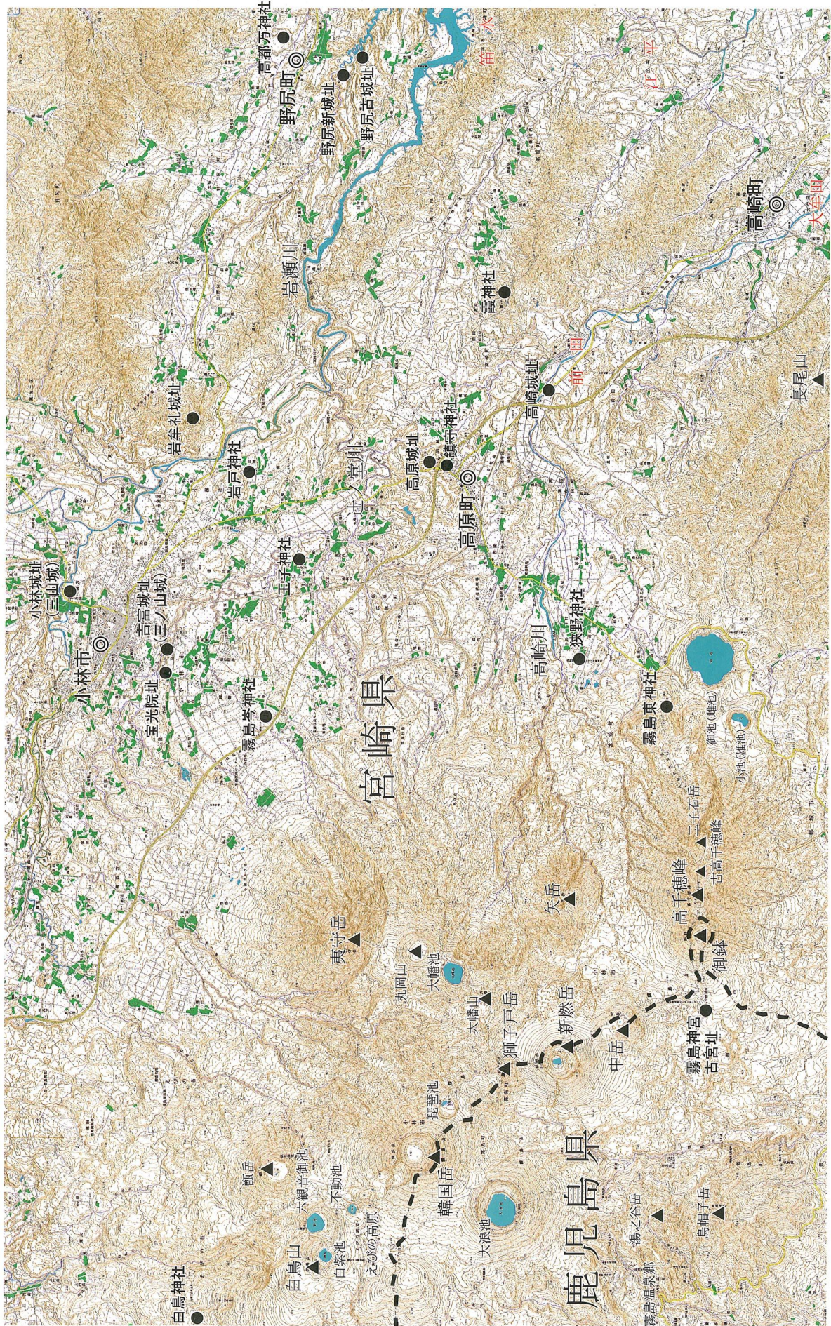
第1図 霧島火山群及び周辺地形図・遺跡位置図
